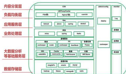
市场及服务网点精细化监控平台系统架构图
